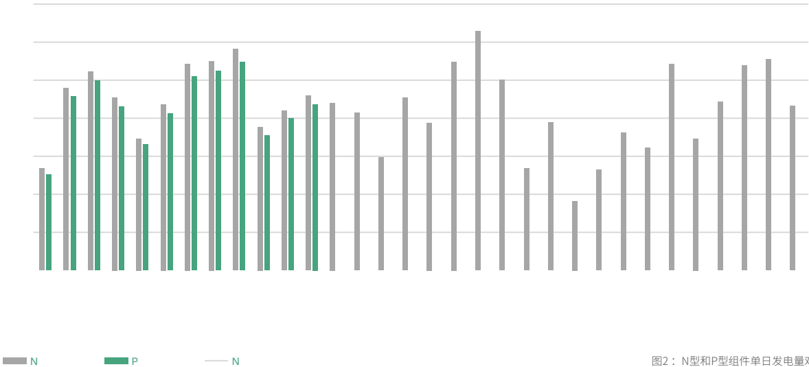
图2：N型和P型组件单日发电量对比
